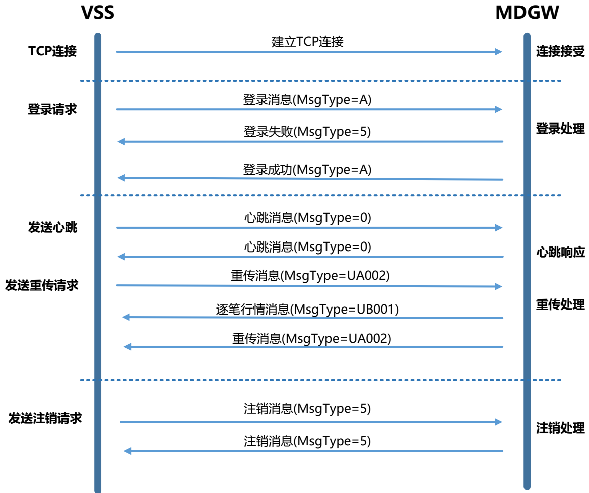
STEP 协议交互图（重传消息）
