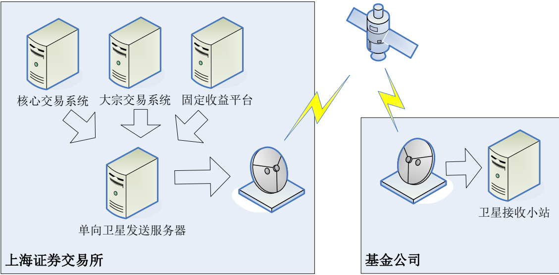
图 4：基金公司接口物理架构
