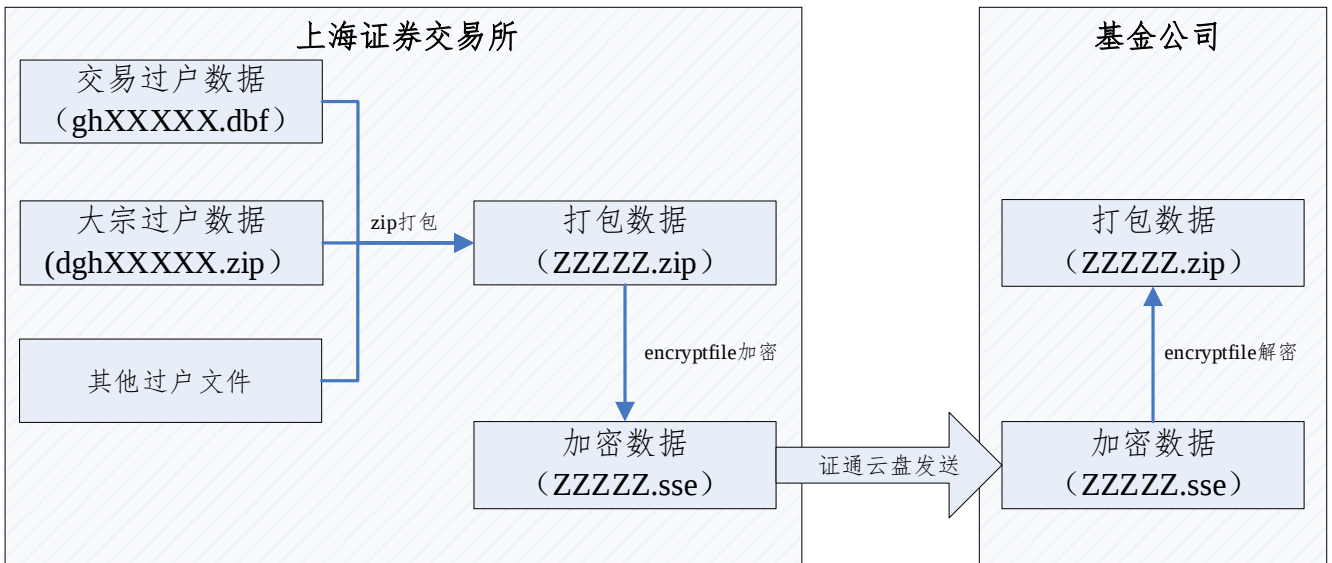
图 2：基金公司接口数据流图
