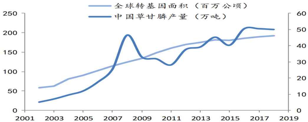
全球草甘膦产量与转基因种植面积相关系数
