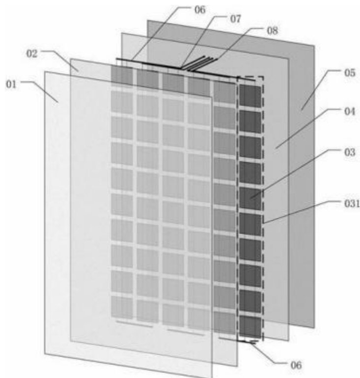
双面双玻电池组件结构图
