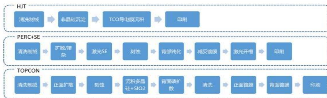
HJT 电池及其他电池生产工艺流程对比图
