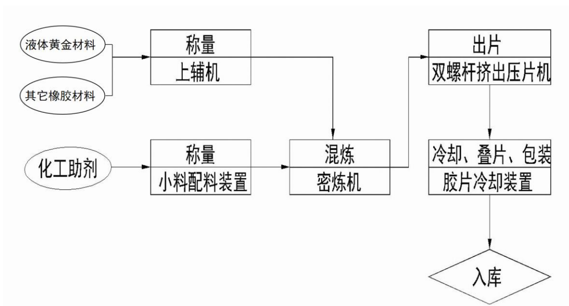
图 4.2-1 生产工艺流程图
