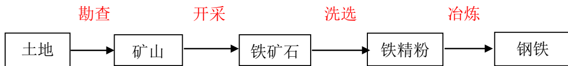
图表 1 铁矿石采选加工程序
