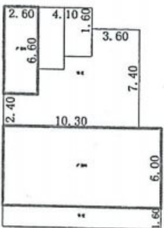
五层平面图
