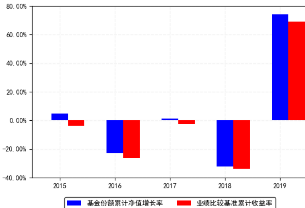
南方中证500信息技术ETF每年净值增长率与同期业绩比较基准收益率的对比图
