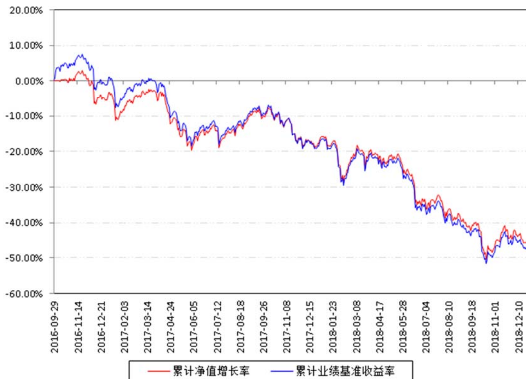
南方中证1000ETF累计净值增长率与同期业绩比较基准收益率的历史走势对比图
